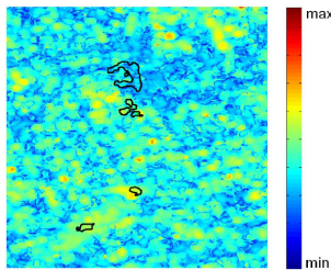
FIG. 5: image du double-rebond, obtenue par un paramètre issu d'une décomposition polarimétrique de Yamaguchi
