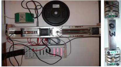
Figure 1 : Le robot expérimental et l'accouplement flexible
